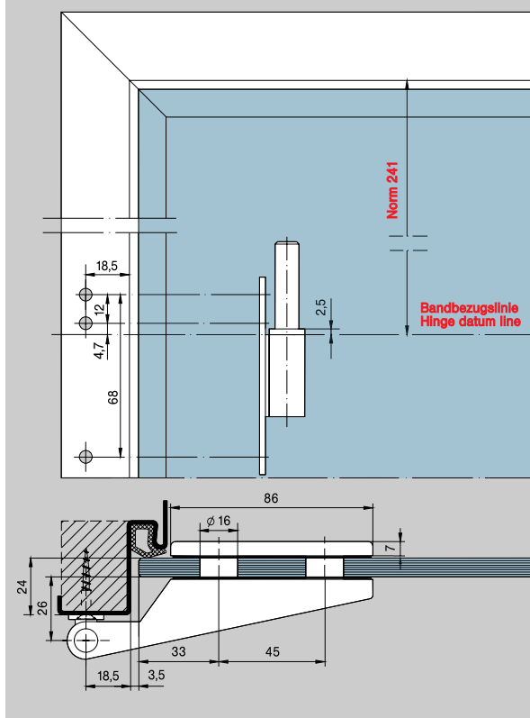
Aufsraub-Rahmenteil
